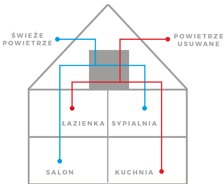
SCHEMAT DZIAŁANIA
